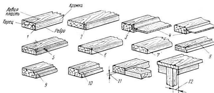
Рис. 4. Элементы составных частей мебельных изделий: 1 - брус, 2 - раскладка, 3 - штапик, 4 - филленка, 5 - фаска, 6 - смягчение, 7 - закругление, 8 - галтель, 9 - калевка, 10 - фальц, 11 - платик, 12 - свес
